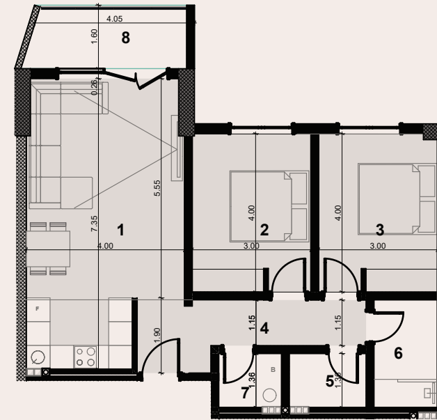
Lamela A1-A4 | Tipi - A2 | KATI 1,5,9 | S= 88.12m2
